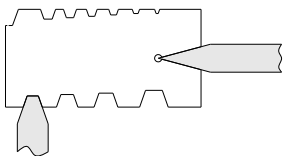
刀头角度、尺寸对比检测
