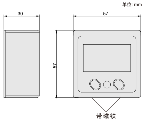
用作倾角仪
