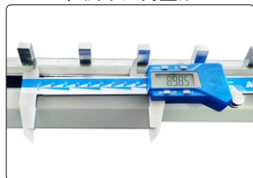
检测卡尺内量爪
