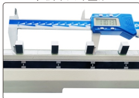
检测卡尺外量爪
