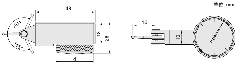
单位: mm
