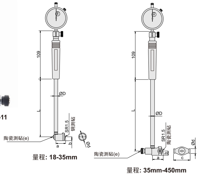
215系列(选配)
