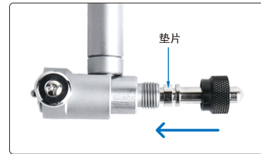
测头安装
