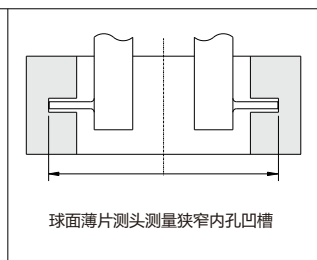
测量内凹槽和外凹槽
