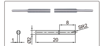
球面薄片长测头(标配)
