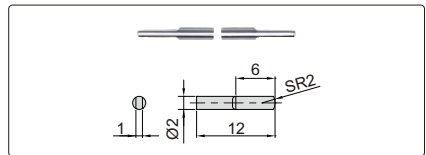
球面薄片测头(标配)
