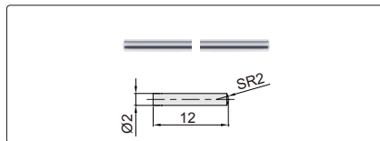
球面/平面长测头(标配)
